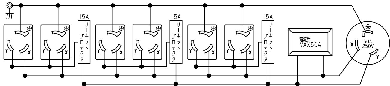
内部配線図
